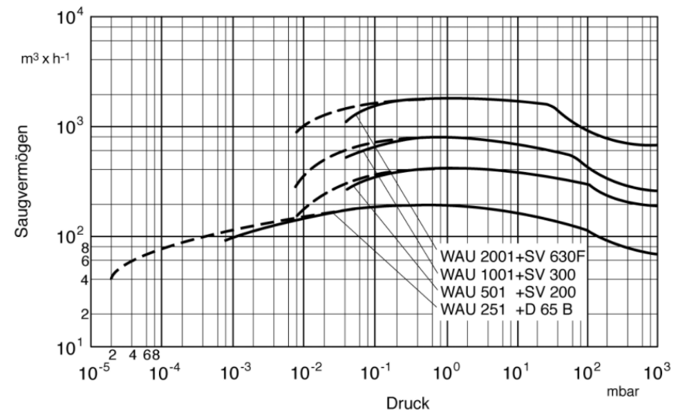
Saugvermögenskurve
