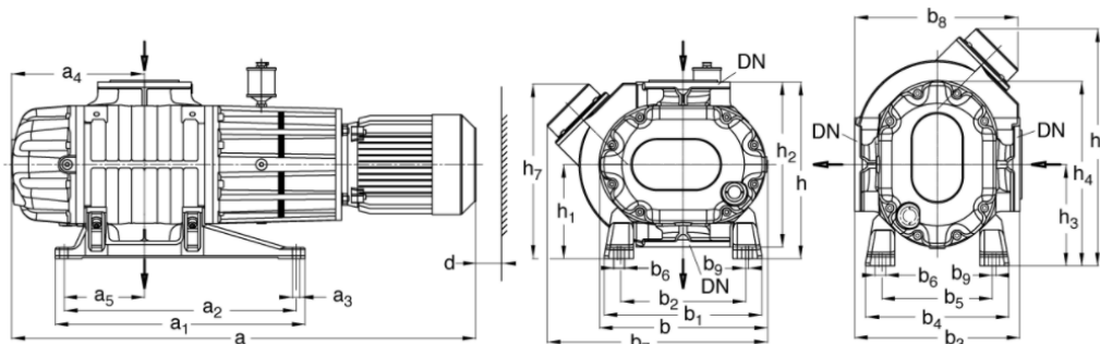
Maßzeichnung
